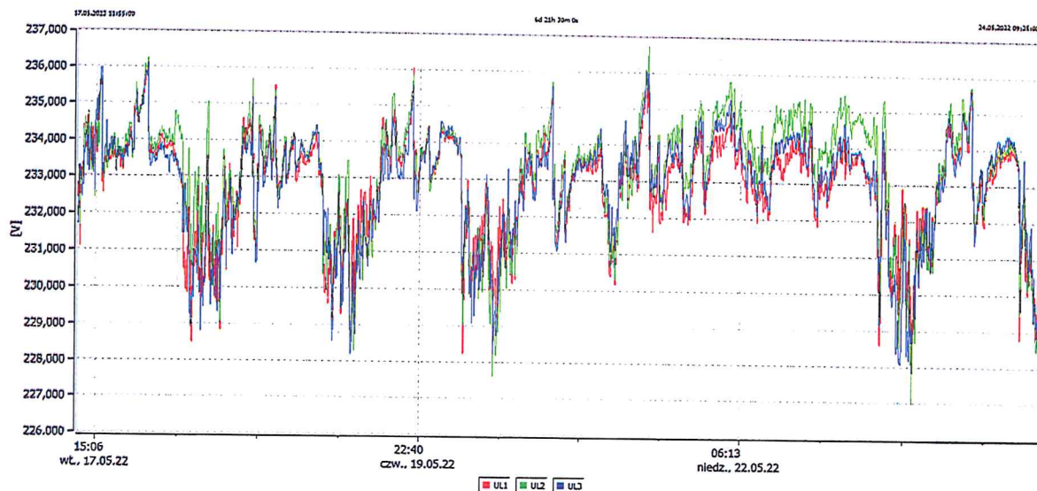
Wykres 1. Napięcie skuteczne średnie
