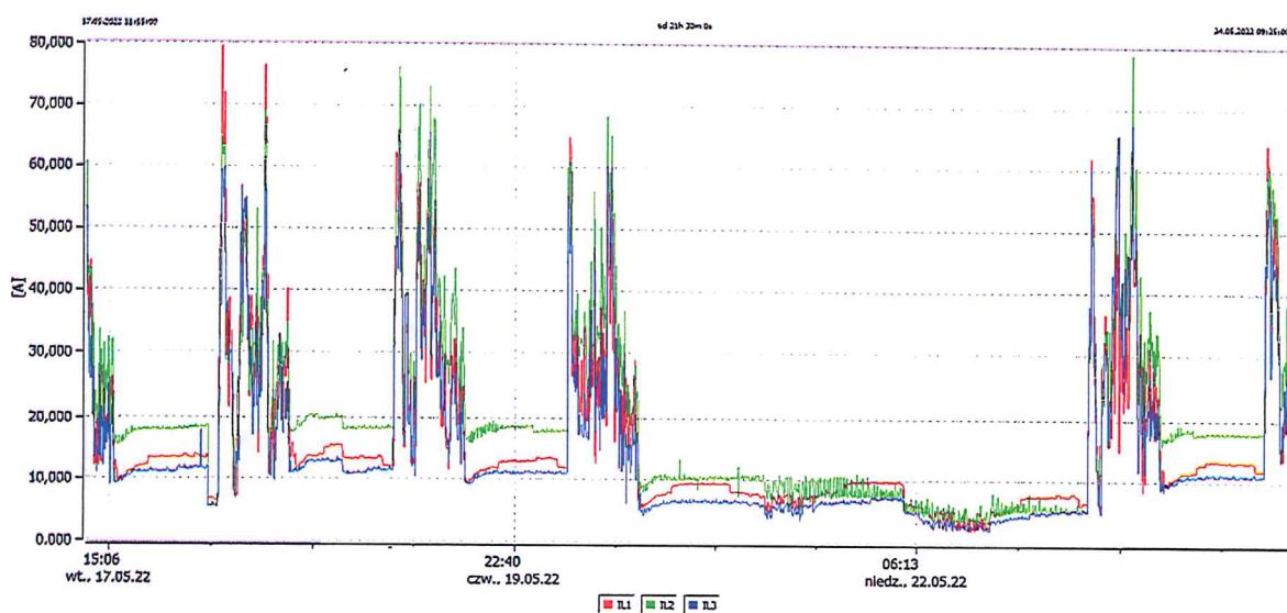
Wykres 2. Prądy skuteczne średnie
